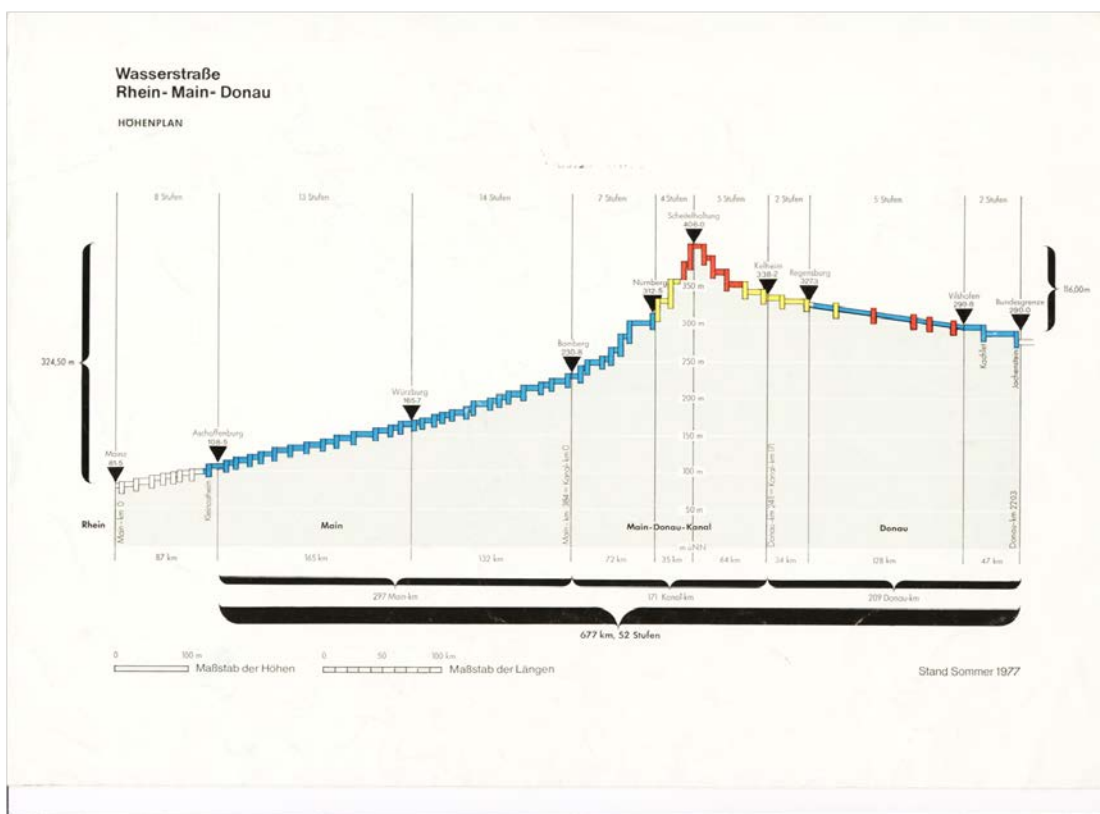
Rajna-Majna-„Duna-Majna Európa-csatorna”- Duna nemzetközi víziút-hálózat áttekintő térképe és hossz-szelvénye / víz-, és energiatakarékos zsilip-rendszer ötlet és terv: Dr. Mosonyi Emil
