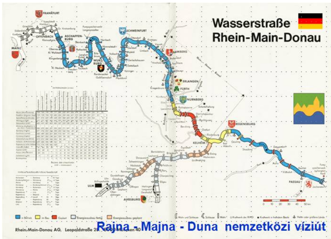
Rajna-Majna-„Duna-Majna Európa-csatorna”- Duna nemzetközi víziút-hálózat áttekintő térképe és hossz-szelvénye / víz-, és energiatakarékos zsilip-rendszer ötlet és terv: Dr. Mosonyi Emil
